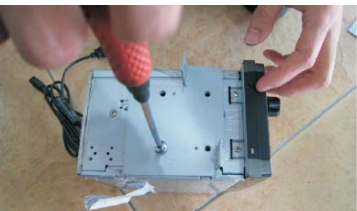
10 将拆下的CD机左右安装支架装在DVD导航上
