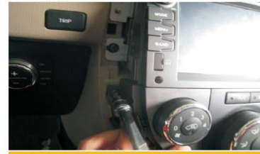
21 打紧固定空调控制面板的四个螺丝
