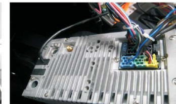
12 插上电源线，收音天线插头和GPS天线插头
