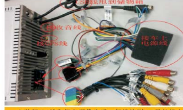
24 装好GPS线和倒车摄像头后，把线接到DVD导航机上再把转接线接好，把USB线引到副驾驶位储物箱位
